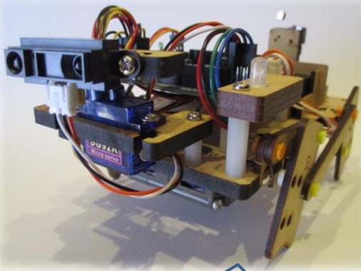
4足歩行ロボット (Fabwalker)
